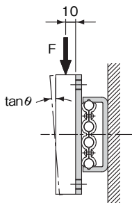
垂直方向负荷
