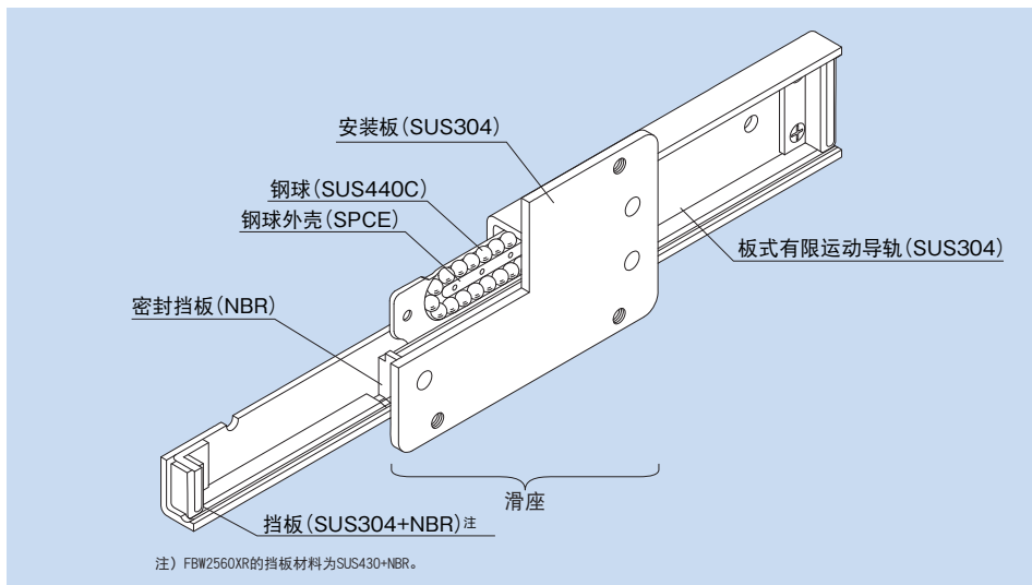
图1 板式导轨FBW-XRUU型的构造
